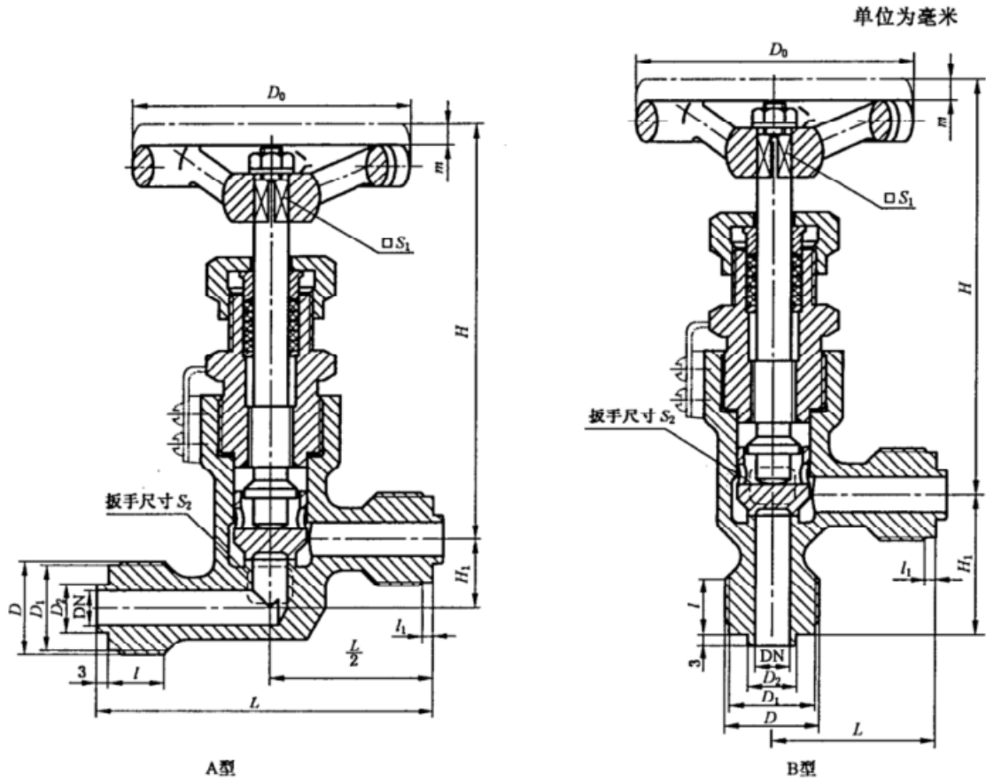
图 1 截止止回阀
